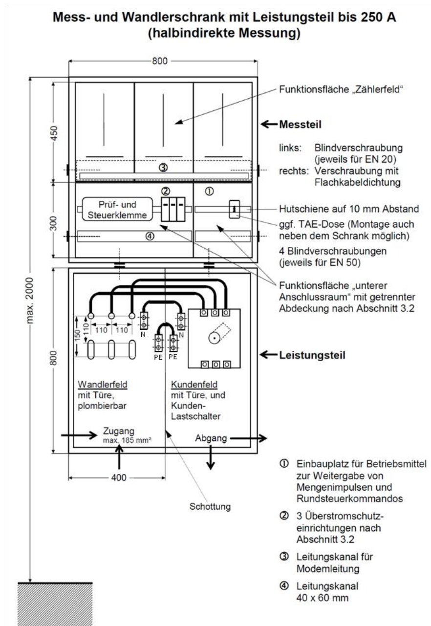
Abbildung: Prinzipieller Aufbau einer halbindirekten Messung (Wandlermessung) bis 250 A
