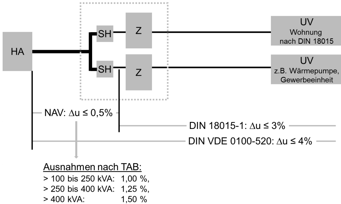
Abbildung: Spannungsfall
